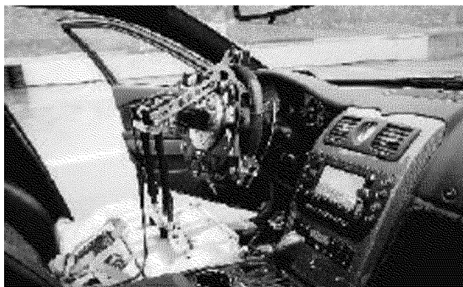
Il sistema di pilotaggio automatico: attuatori azionati da onde radio
